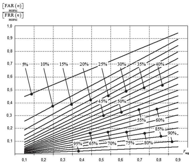
Рис. 4. Отримана нормована залежність співвідношення \frac{[FAR(n)]_{\text{НОРМ}}}{[FRR(n)]_{\text{НОРМ}}} від значення r_{\text{пор}} для досліджуваних зображень (рис. 1)
