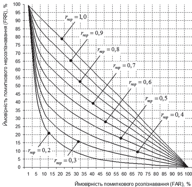
Рис. 3. Отримана залежність між помилками 1-го та 2-го роду при різних r_{\text{пор}} для досліджуваних зображень (рис. 1)
