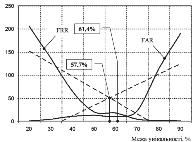
Рис. 5. Відповідність розрахованих співвідношень множин [FRR(n)] та [FAR(n)] загальновідомим даним
