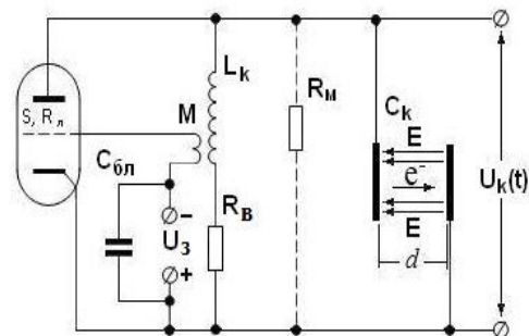
Рис. 8. ВЧ система одиночного резонансного контуру ( L_K , C_K , R_B ) з тріодом ( S , R_n ) де електроди ємкості C_K , розташованих на відстані d , є емітерами електронів ВЕЕ, витрачаючи ВЧ енергію, як активним опором ВЕ мультипакції R_M , що підключається до контуру
