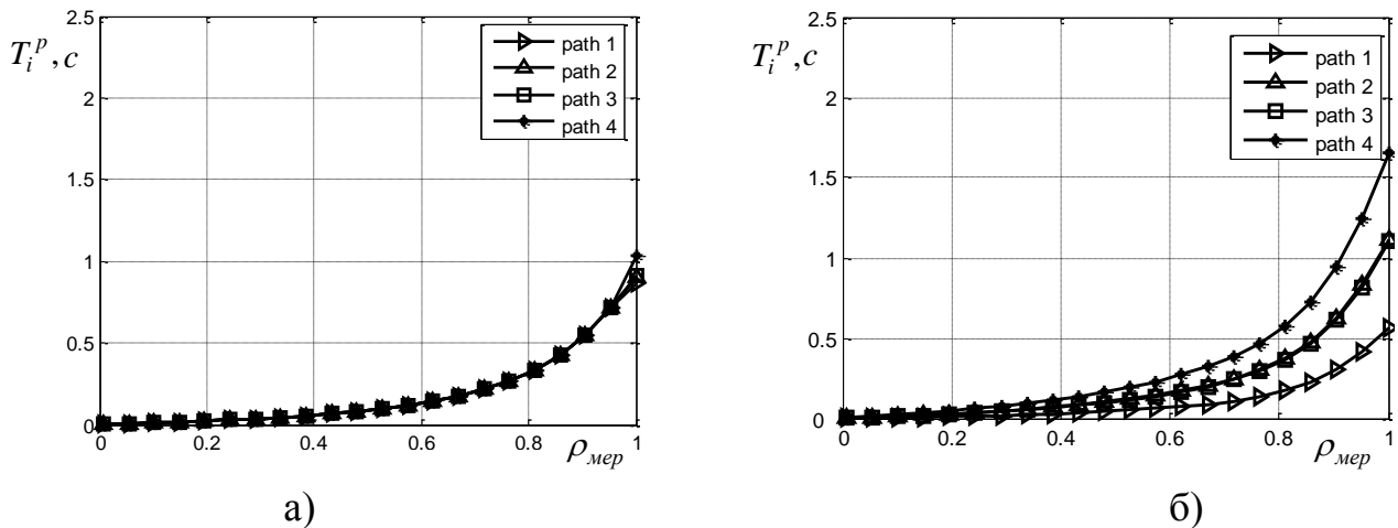
Рис. 7. Середня затримка в окремих маршрутах для тензорної [NP, \pi\omega] -моделі (а) та моделі M3
