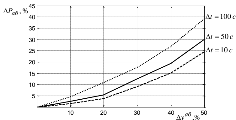
Рис. 9. Залежність втрат продуктивності \Delta P_{a\bar{b}}(\Delta y^{a\bar{b}}) через погрешності в оцінюванні обсягів абонентського навантаження
