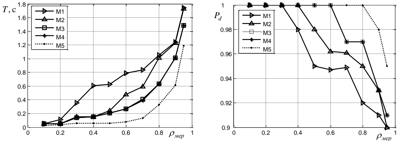
Рис. 6. Результати лабораторного дослідження тензорної [NP, \pi\omega] -моделі ТКС (M5) у порівнянні з іншими потоковими моделями ТКС (M1) – (M4)
