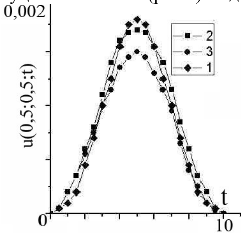
Рис. 5. Зсув у центрі пластини при різному кроці просторової змінної. 1. \Delta x = \frac{1}{15} , 2. \Delta x = \frac{1}{12} , 3. \Delta x = \frac{1}{8} .
