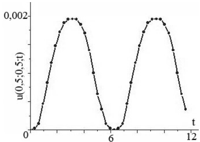
Рис. 2. Зсув при навантаженні q(x,t) = q_0 \sin t .
