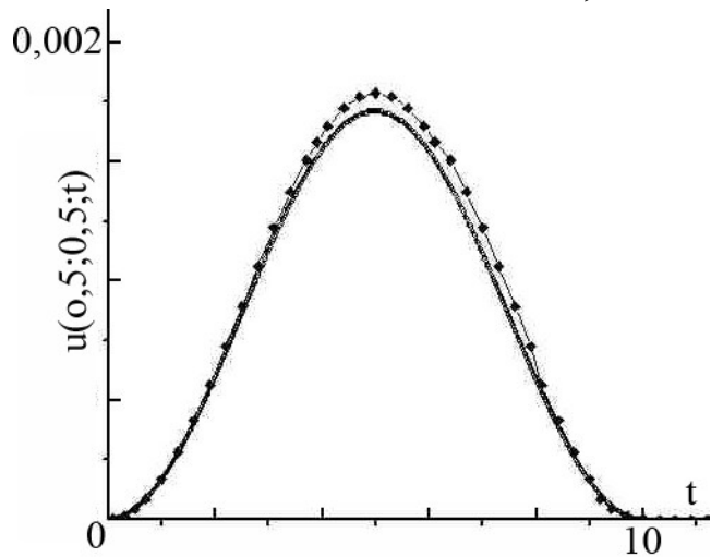
Рис. 6. Порівняння результатів для першої основної задачі.
