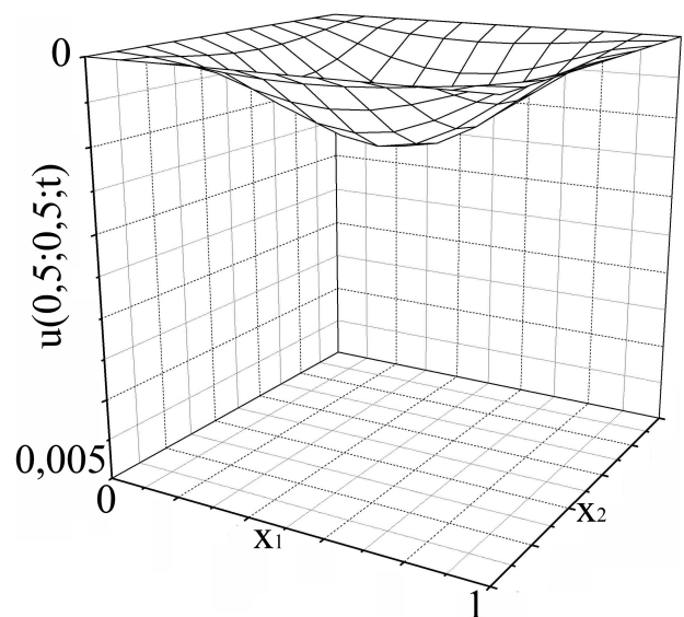
Рис. 4. Форма серединної площини пластини t = 4c .
