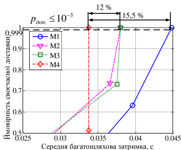
в) за ймовірністю своєчасної доставки при інтенсивності потоку, що надходить до мережі, 200 1/с
