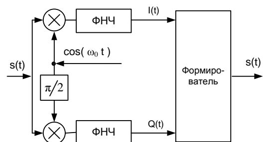
Рис. 10. Демодулятор КАМ
