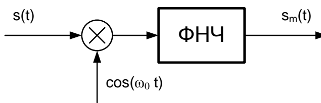
Рис. 4. Демодулятор АМ
