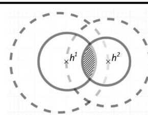
Рис. 1 Схеми класифікації для двох класів: суцільна лінія – межа околу, пунктирна – межа класів
