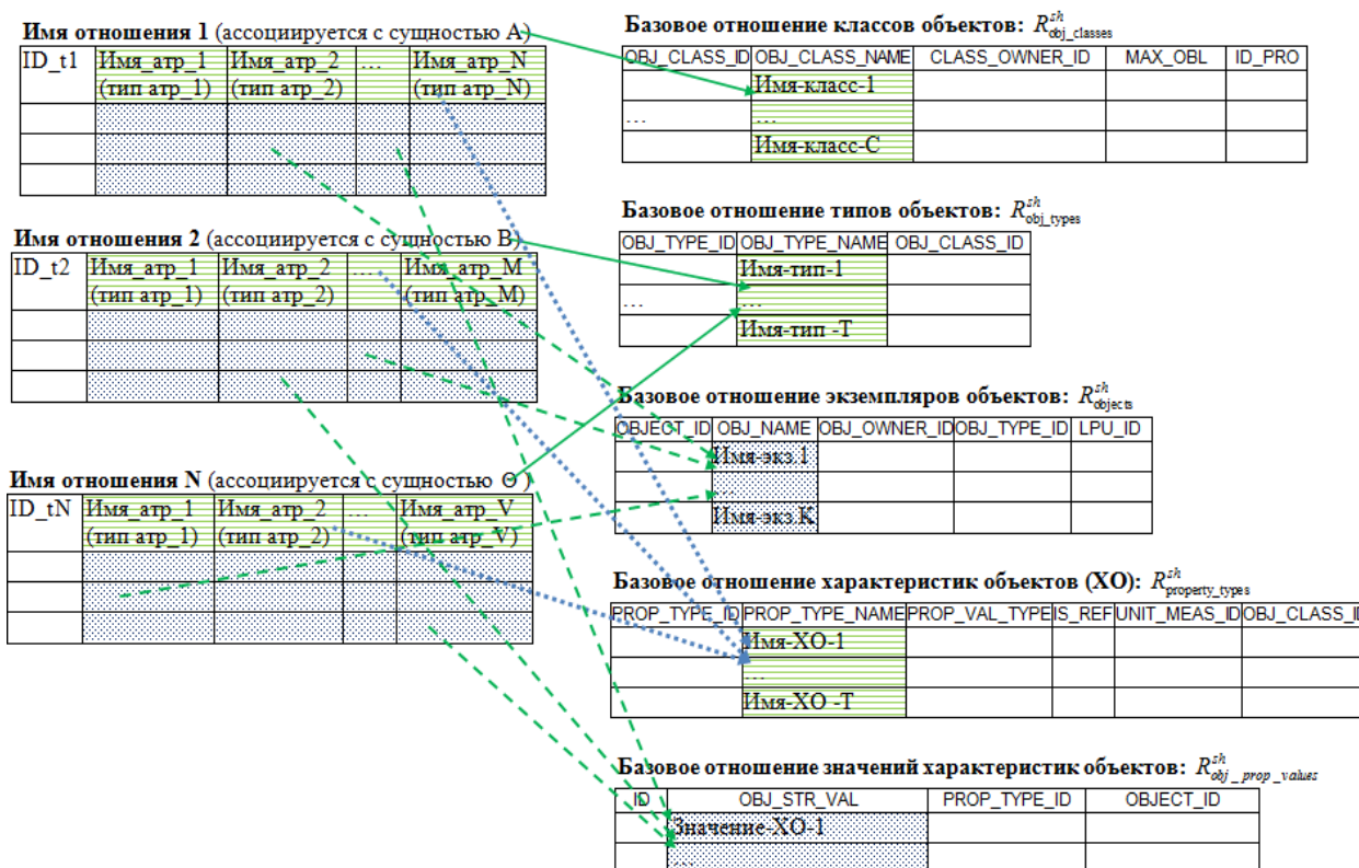
Рис. 3. Схематичное представление трансформации описания предметной области в инвариантную к ПрО схему БД и в схему РБД, спроектированную по традиционной технологии
