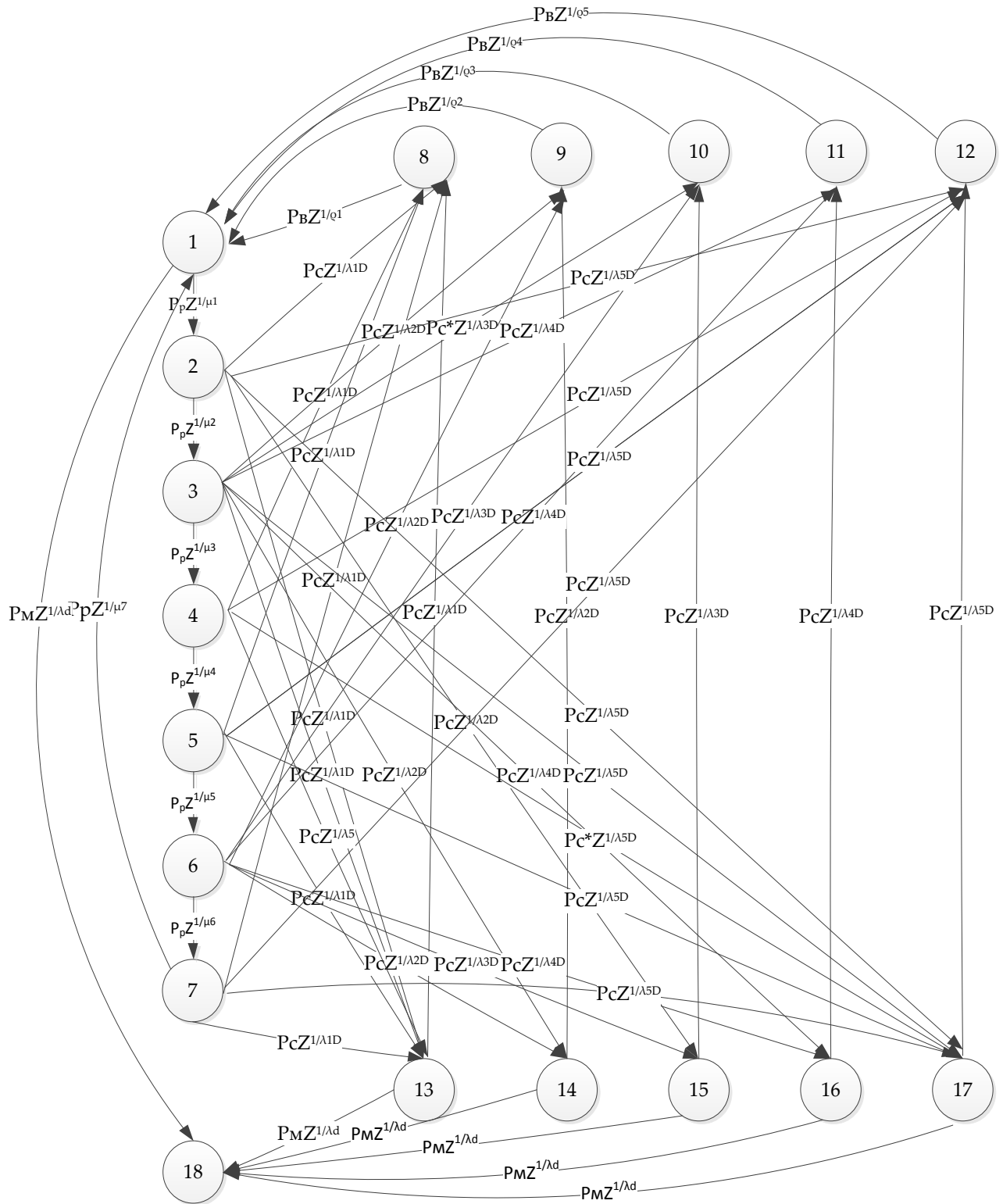
Рис. 2. Вероятностно-временной граф функционирования системы сетевого управления на основе WBEM
