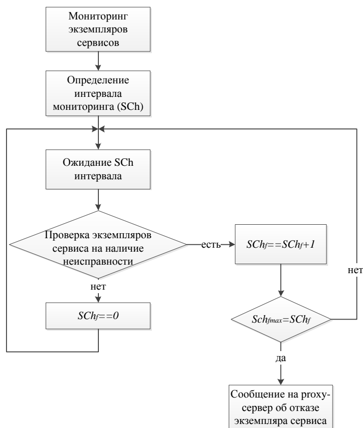
Рис. 1. Алгоритм мониторинга экземпляров сервисов
