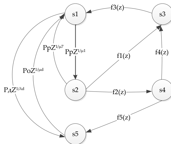
Рис. 3. Промежуточные преобразования вероятностно-временного графа функционирования системы сетевого управления на основе WBEM
