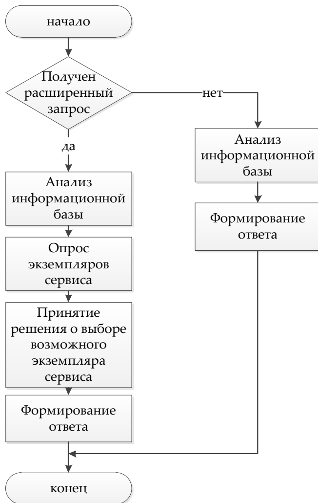
Рис. 7. Алгоритм работы системы мониторинга при выборе экземпляра сервиса
