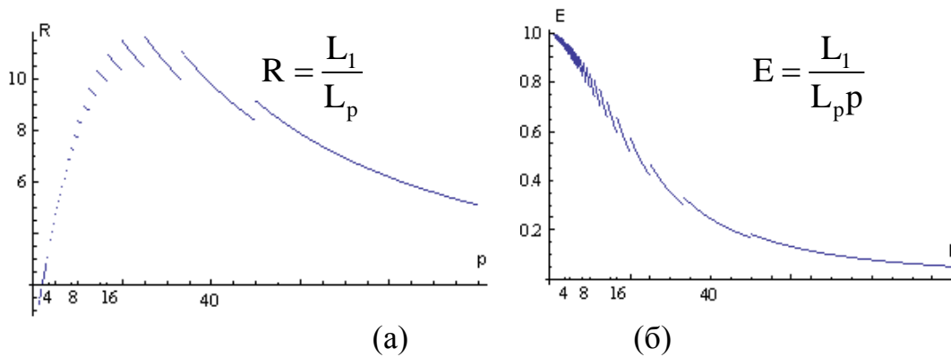
Рисунок 1. Графики ускорения (а) и эффективности (б)
