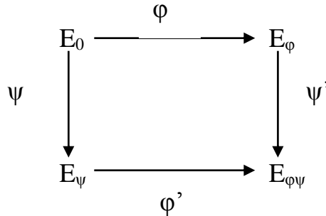
Рисунок 1.1 - Спрощена схема криптоперетворень на ізогеніях ЕК
