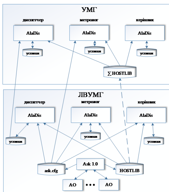
Рис.1. Структурна схема організації аналізу газовимірювальної інформації
