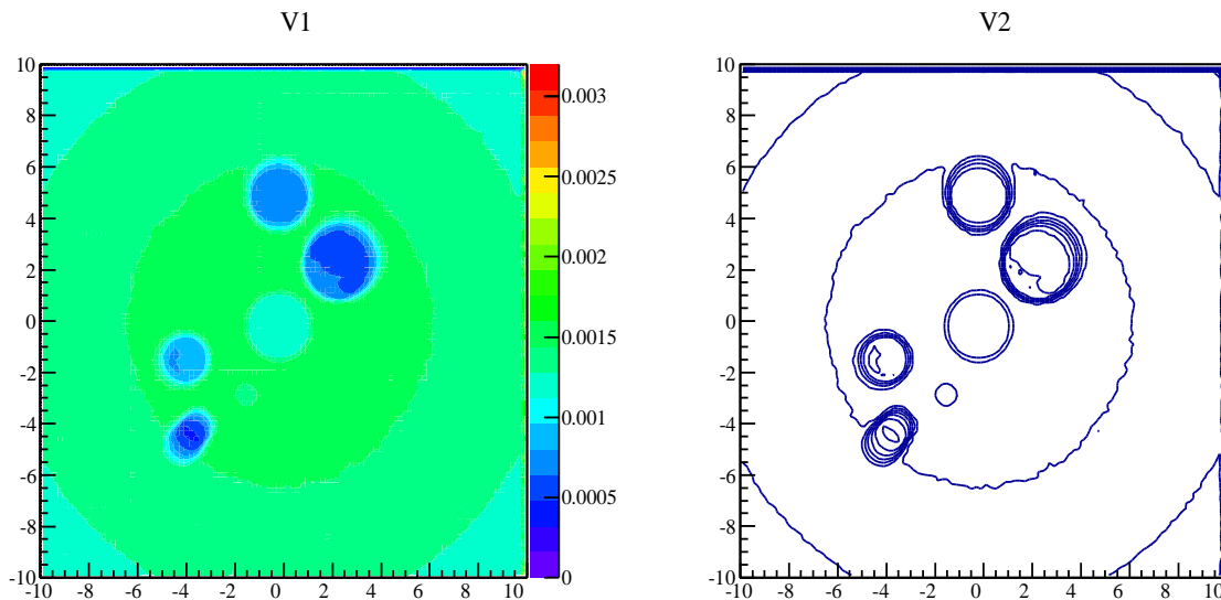
Рис. 3. Результати моделювання зборки при опроміненні нейтронами на виході з системи формування НР-установки
