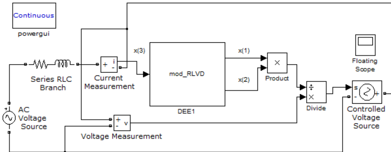
Рис. 1. Вигляд візуально-блокової моделі комплексу «РЛВД – дросель», реалізованої в Simulink
