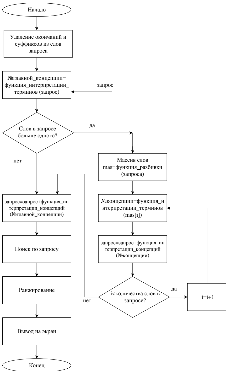
Рис.1. Алгоритм поиска данных по онтологической модели
