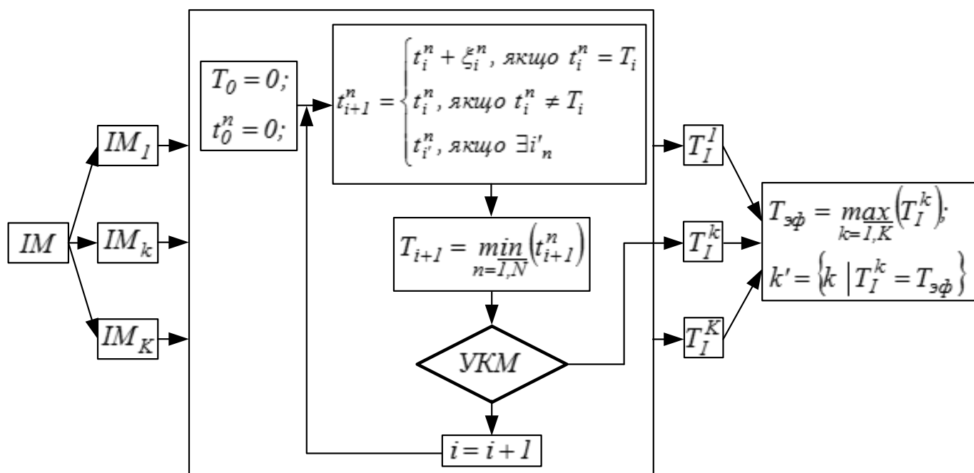
Рисунок 2 – Метод порівняння ефективності розподілених імітаційних моделей за максимальним просуванням модельного часу
