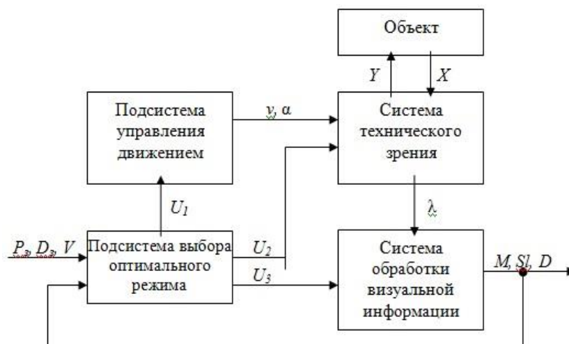
Рис. 1. Модель адаптивной системы управления для мобильного робота
