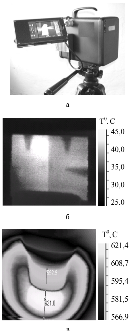
Рис.4. Внешний вид АТП с КПК (а); выявление дефектов в слоистых материалах: приемник – КРТ линейка (б); контроль температурных полей при выращивании монокристаллов CsI: момент касания затравки с расплавом (в)
