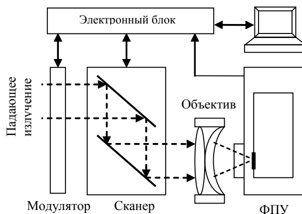
Рис. 1. Блок-схема АТП
